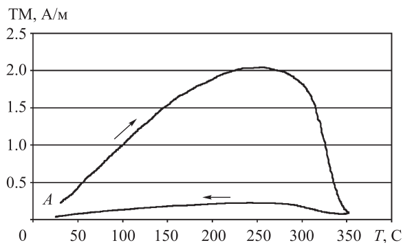
Рис. 4. Изменение намагниченности образца 29/1(2) из нулевого состояния A при нагреве и охлаждении в отсутствие поля. Нулевое состояние A было получено при размагничивании ПТОН ( 350\text{--}300^\circ\text{C} , 0.1 мТл) переменным магнитным полем h \approx 0.1 Тл
