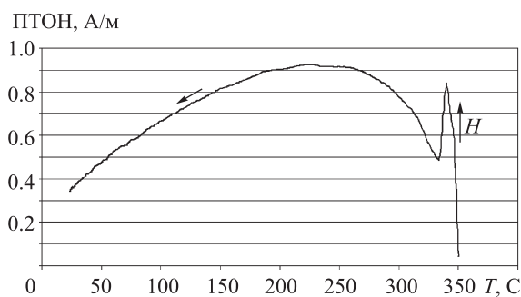
Рис. 5. Образование ПТОН на образце 29/1(2) в интервале T = 350\text{--}340^\circ\text{C} в H = 0.1 мТл и в интервале T = 340\text{--}20^\circ\text{C} , H = 0.11 мТл
