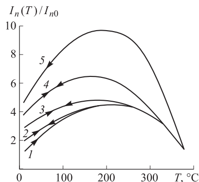
Рис. 7. Циклическое размагничивание I_n образца переходного базальта [9]
