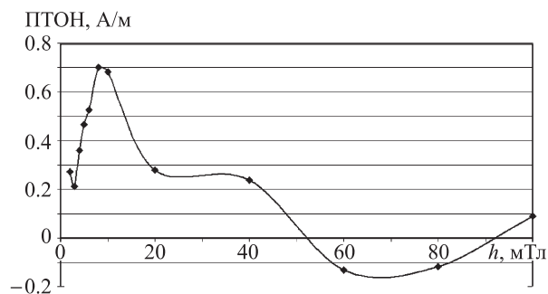
Рис. 6. Размагничивание ПТОН ( T = 325\text{--}300^\circ\text{C} , H = 0.1 мТл) образца 16/30 переменным полем
