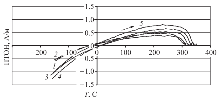
Рис. 3. Изменение ПТОН ( H = 0.1 мТл), созданных в разных температурных интервалах, при нагреве образца 29/1(2) в отсутствие поля: T = 300\text{--}275^\circ\text{C} (1), 310\text{--}300^\circ\text{C} (2), 320\text{--}310^\circ\text{C} (3), 330\text{--}320^\circ\text{C} (4), 340\text{--}330^\circ\text{C} (5)
