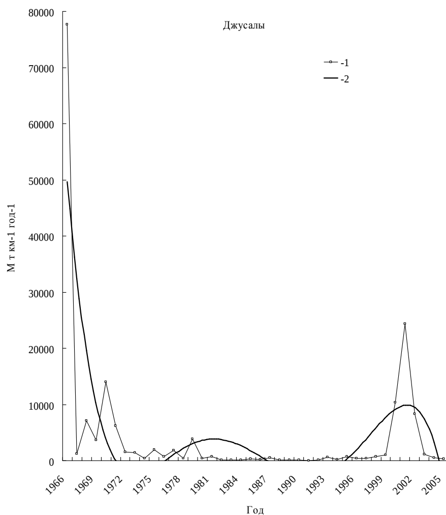
Рис. 7. Многолетний ход массы песка, переносимого пыльными бурями и поземками и сглаженная кривая на метеостанции Джусалы.
