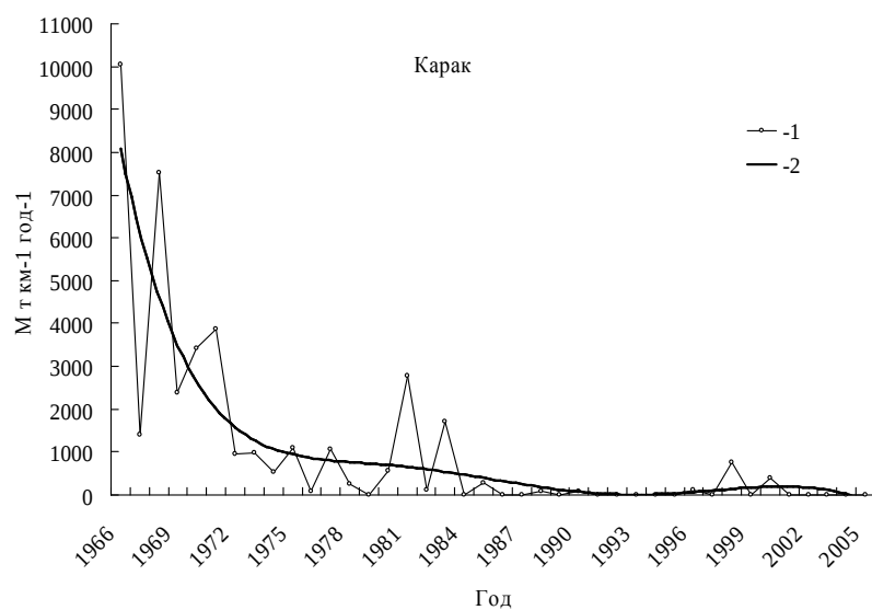
Рис. 6. Многолетний ход массы песка, переносимого пыльными бурями и поземками и сглаженная кривая на метеостанции Карак.
