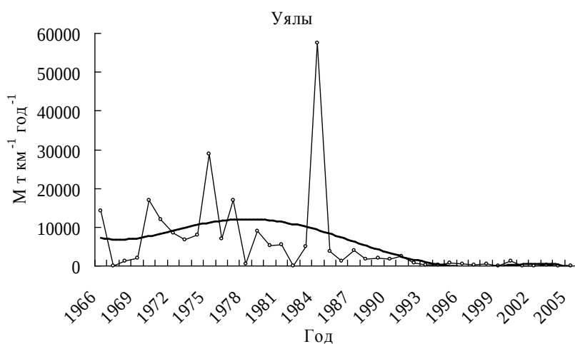
Рис. 2. Многолетний ход массы песка, переносимого пыльными бурями и поземками и сглаженная кривая на метеостанции Уялы.
