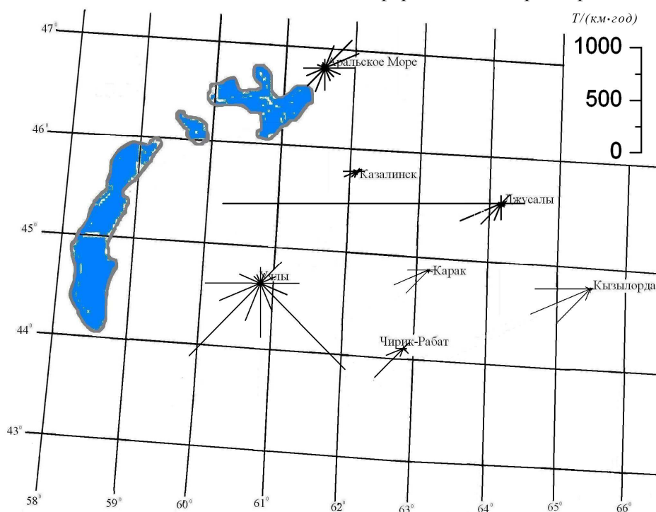
Рис. 8. Многолетние средние годовые розы векторов переноса массы песка ветром в Приаралье.
