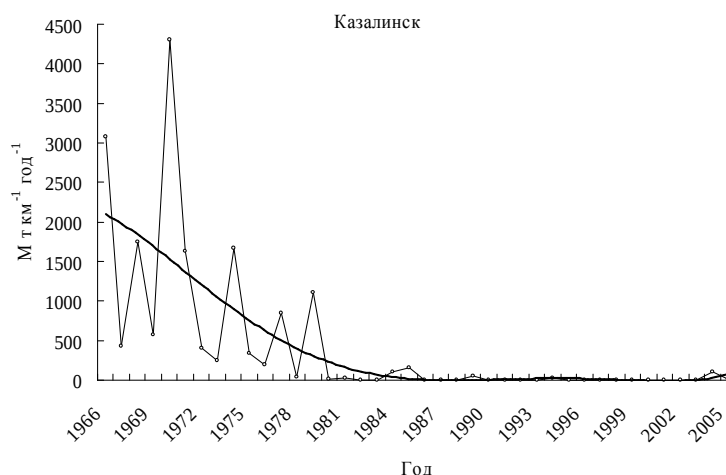
Рис. 3. Многолетний ход массы песка, переносимого пыльными бурями и поземками и сглаженная кривая на метеостанции Казалинск.
