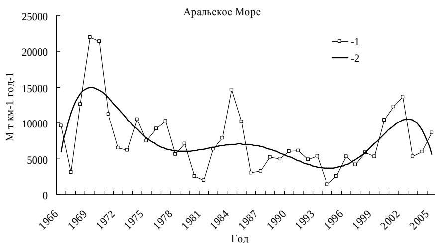
Рис. 1. Многолетний ход массы песка, переносимого пыльными бурями и поземками (1) и сглаженная кривая (2) на метеостанции Аральское Море.
