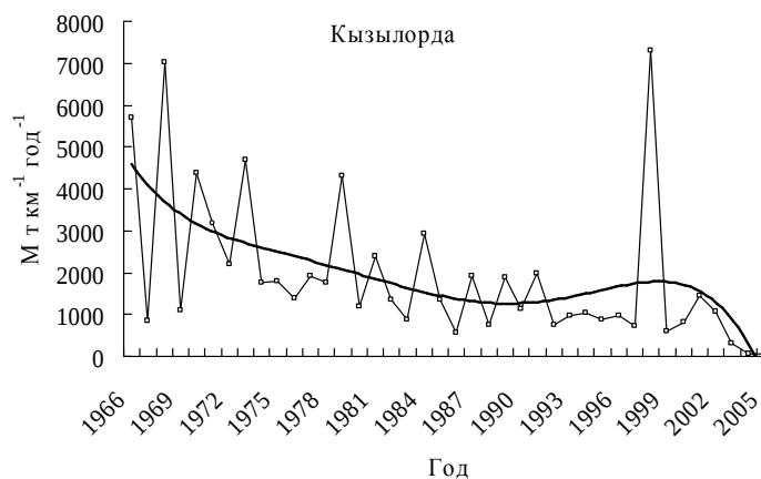
Рис. 4. Многолетний ход массы песка, переносимого пыльными бурями и поземками и сглаженная кривая на метеостанции Кызылорда.
