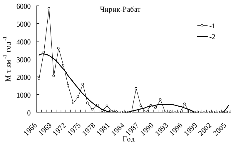
Рис. 5. Многолетний ход массы песка, переносимого пыльными бурями и поземками и сглаженная кривая на метеостанции Чирик-Рабат.
