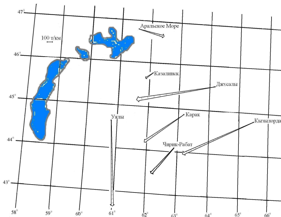
Рис. 9. Многолетние средние годовые результирующие векторы переноса песка ветром в Приаралье.
