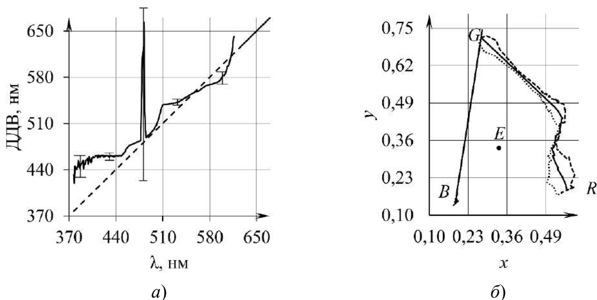
Рис. 4. а) спектральная зависимость ДДВ в случае идеальной цветопередачи (пунктирная линия) и экспериментально полученная (сплошная линия). Величина СКО нанесена знаком «I»; б) экспериментально определенный цветовой охват камеры Canon EOS 500D на диаграмме ( x, y )
