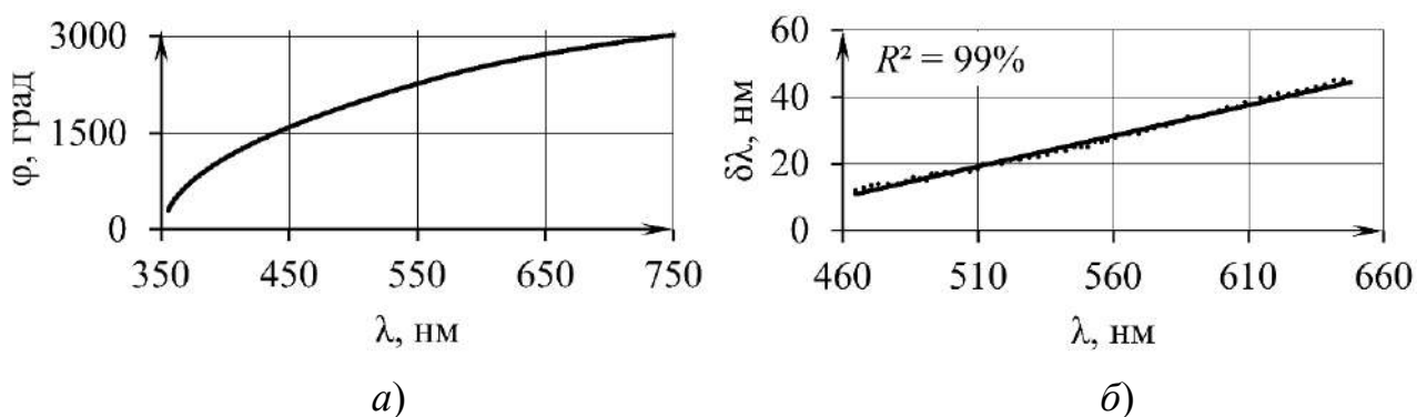
Рис. 2. К градуировке монохроматора:
