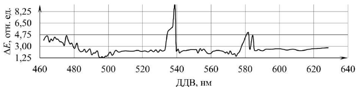
Рис. 6. Компьютерное зрение. Спектральное распределение \Delta E для пар стимулов, отстоящих друг от друга на величину \Delta \lambda = 1 \pm 0,25 нм
