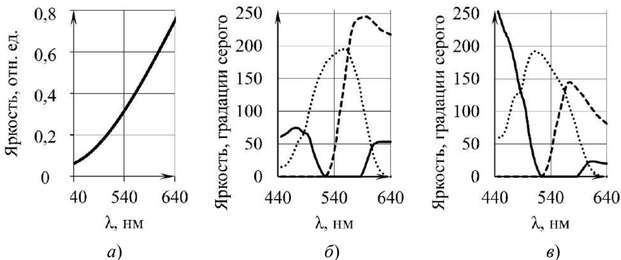
Рис. 3. а ) Фрагмент спектра источника излучения К220-100; б ) спектральный отклик каналов RGB , полученный непосредственным фотографированием; в ) спектральный отклик каналов RGB после деконволюции со спектром лампы
