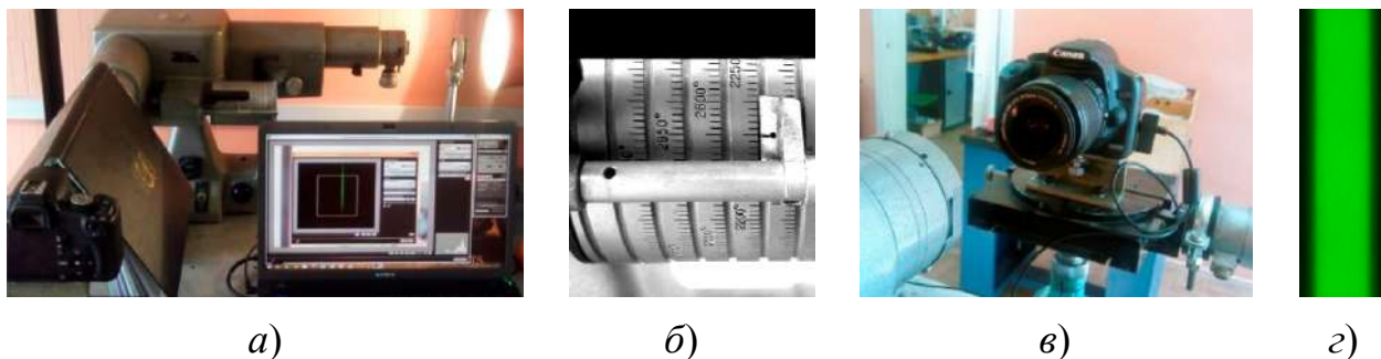
Рис. 1. а) фотография экспериментальной установки; б) фотография барабана длин волн; в) фотография камеры с объективом в сборке; г) фотография фрагмента выходной щели
