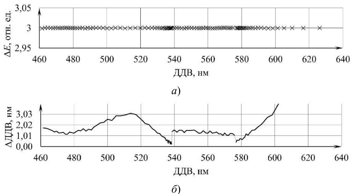
Рис. 5. Компьютерное зрение:
