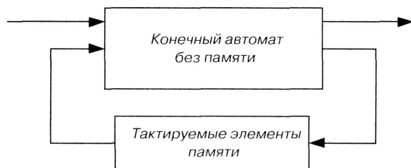
■ Рис. 1. Синхронный автомат с памятью
