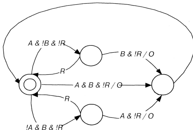
■ Рис. 4. Автомат Мили для решения задачи АВРО
