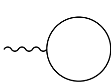
Figure 4 – One external photon Рис. 4 – Один внешний фотон Слика 4 – Један спољашњи фотон
