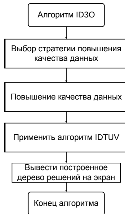
Рисунок 1. Алгоритм ID3O
