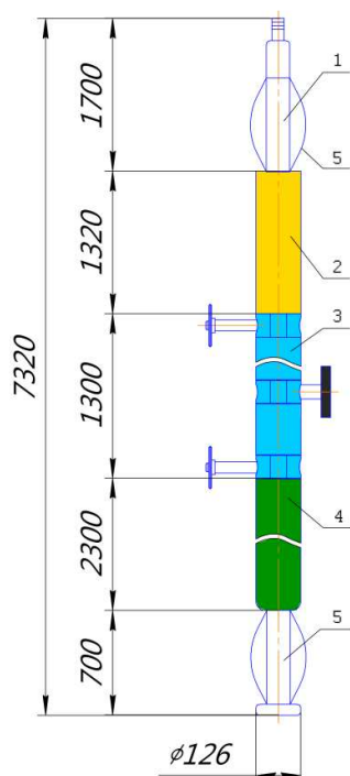
Рис. 2. Компоновка пластоиспытателя:
