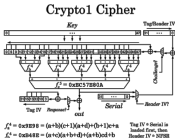
Рис. 10. Алгоритм Crypto 1
