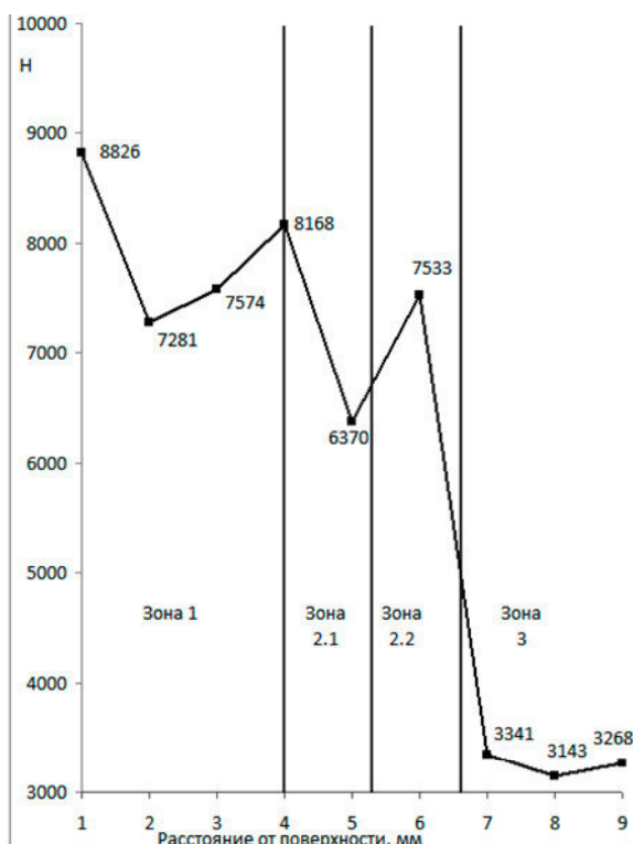
Рис. 3. Изменение твердости по Виккерсу от поверхности при наплавке проволокой Нп-30ХГСА с добавкой порошка ПГ-10Н-01: 1 – зона наплавки; 2 – зона термического влияния: 2.1 – зона легирования; 2.2 – зона термического воздействия; 3 – основной металл
