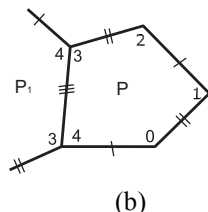
Рис. 5. К лемме 5
