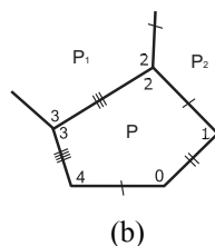
Рис. 4. К лемме 4
