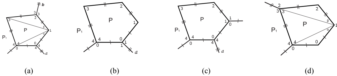
Рис. 9. К лемме 8
