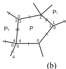
Рис. 6. К лемме 6
