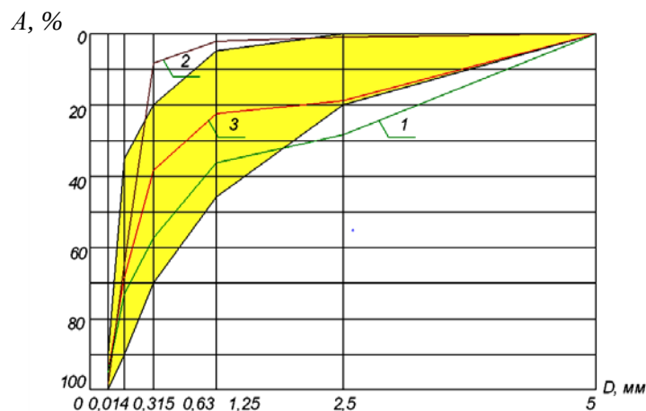
Рис. 1. Зерновой состав заполнителей: 1 – отсевов гранитного карьера; 2 – днепровского песка; 3 – смеси днепровского песка и отсевов гранитного карьера
