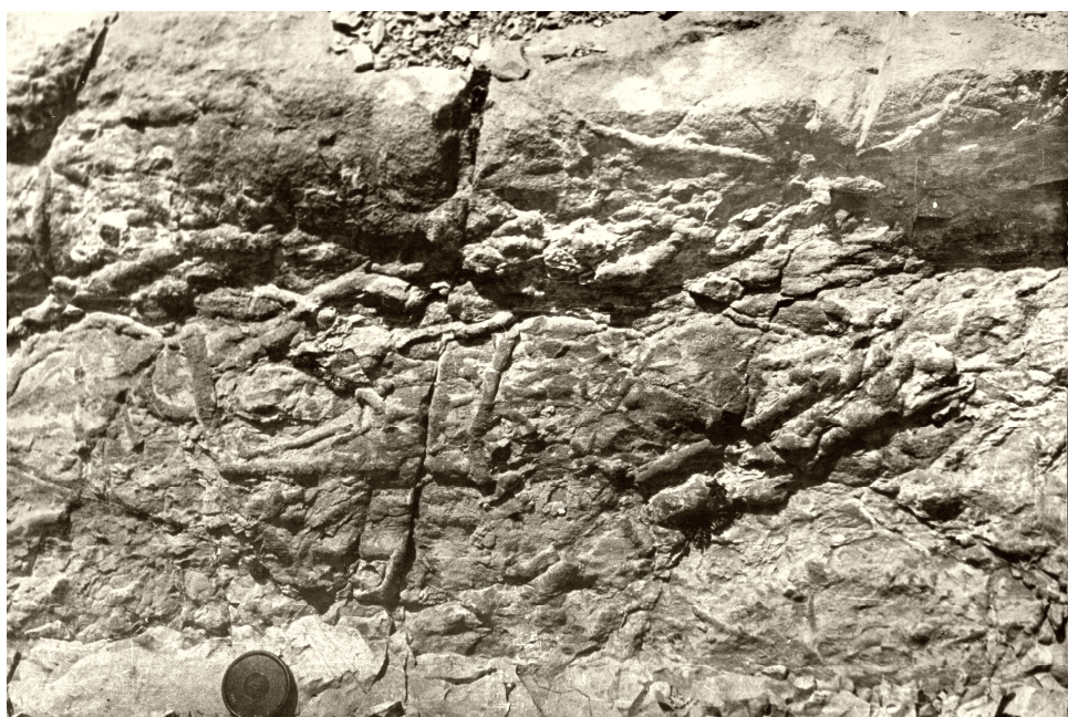
Рис. 10. Слпки ходов илоедов на подошве флишевых ритмов верхнемеловых обломочных известняков. Река п. Дариндересичай, Севанский (Шахдагский) хребет. М. Кавказ.
