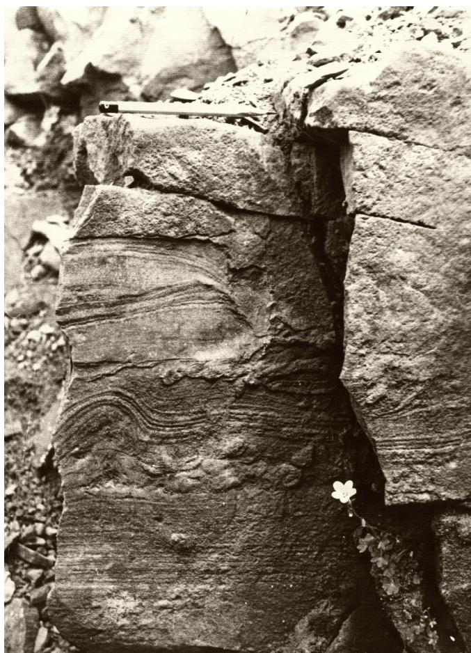
Рис. 9. Классический первый элемент флишевого ритма. Верхнемеловые обломочные известняки. Река п. Дариндересичай, Севанский (Шахдагский) хребет. М. Кавказ. Нижняя часть — прямая градационная слоистость, переходящая в параллельную горизонтальную. Над ней пloyчатый горизонт, указывающий на подводное сингенетическое оползание осадка. Верхняя часть — разнонаправленная косая слоистость.
