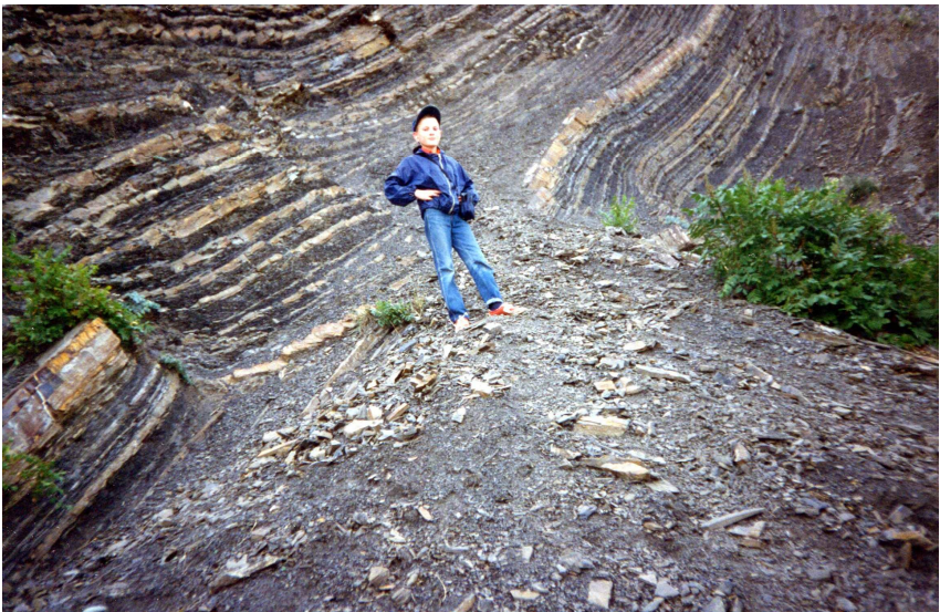
Рис. 5. Обнажение тонкоритмичного флиша таврической серии в береговых обрывах между г. Алуштой и п. Малореченское. Более толстые и светлые слои сложены песчаниками и алевролитами, между ними прослои сиреневато-серых аргиллитов 3 .
